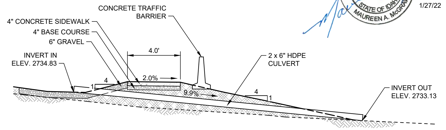
G SECTION G C5 SCALE: 1"=4'-0"
