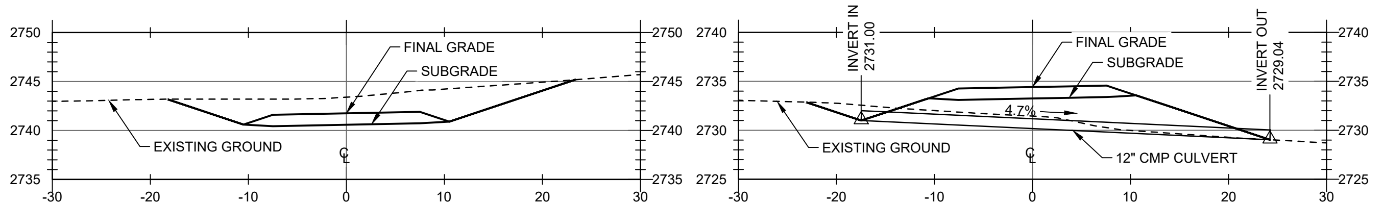
A C2 SECTION STA 0+40 SCALE: 1"=10'
