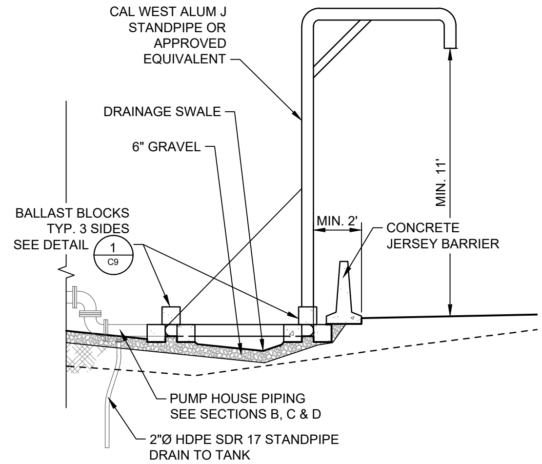
E SECTION E C5,C7 SCALE: 1"=4'-0"
