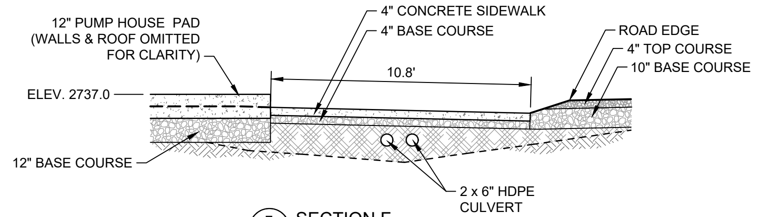
F SECTION F C5 SCALE: 1"=4'-0"
